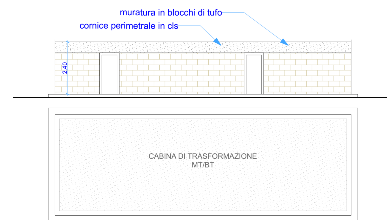
P.01 PIANTE E PROSPETTO TIPO LOCALI TECNICI 1:100
