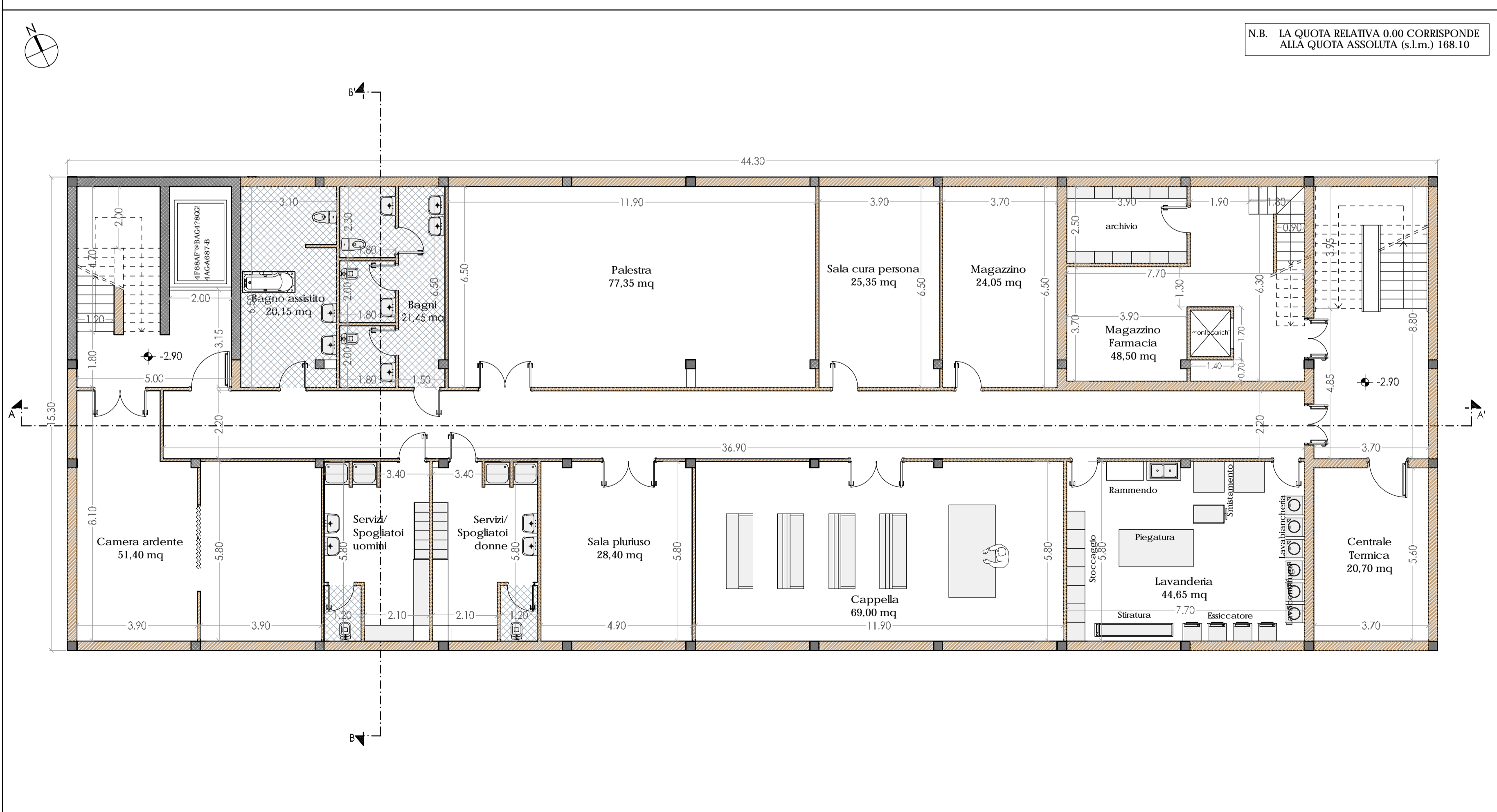
PIANTA PIANO INTERRATO - rapp. 1:100
