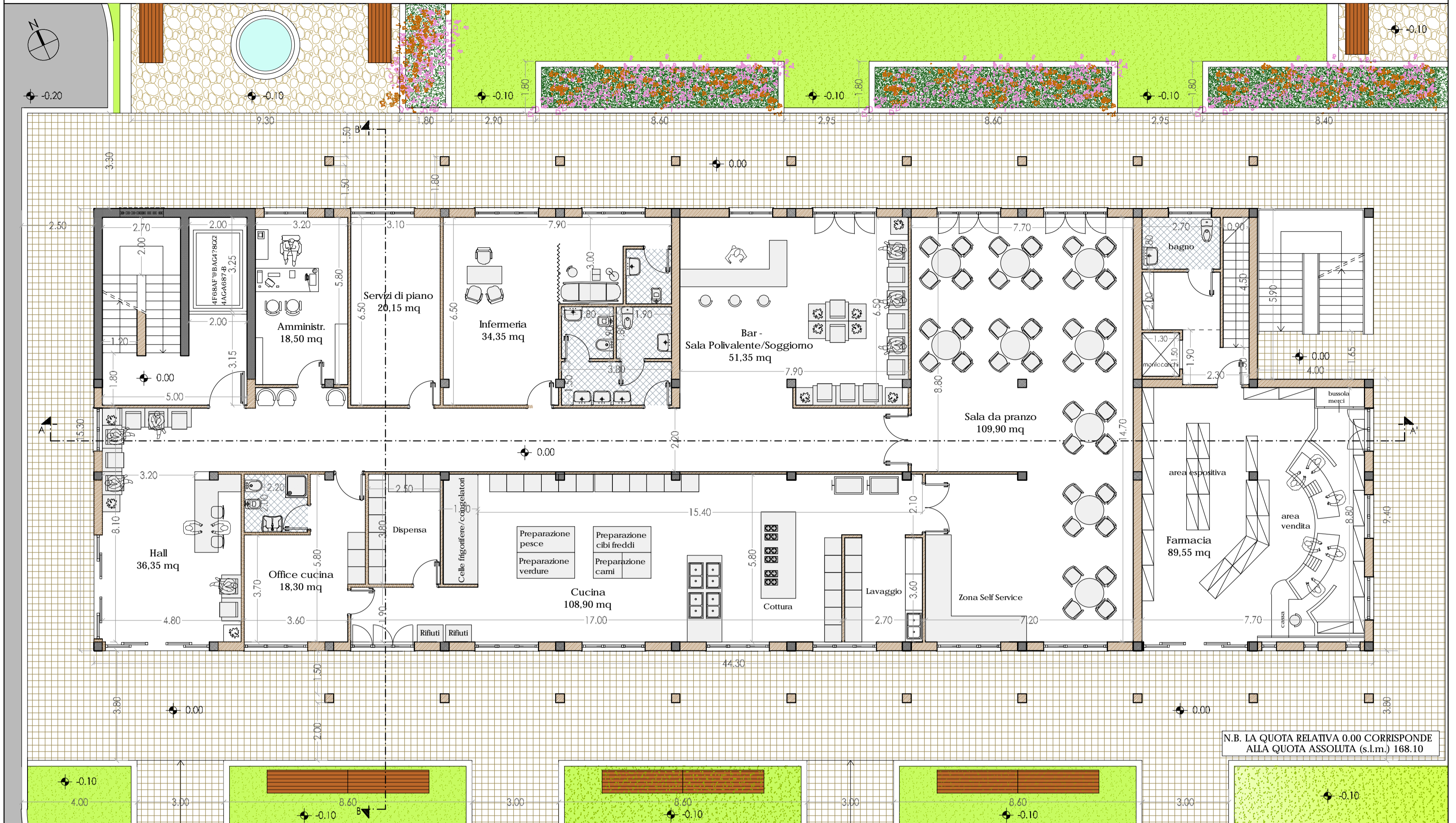
PIANTA PIANO TERRA - rapp. 1:100
