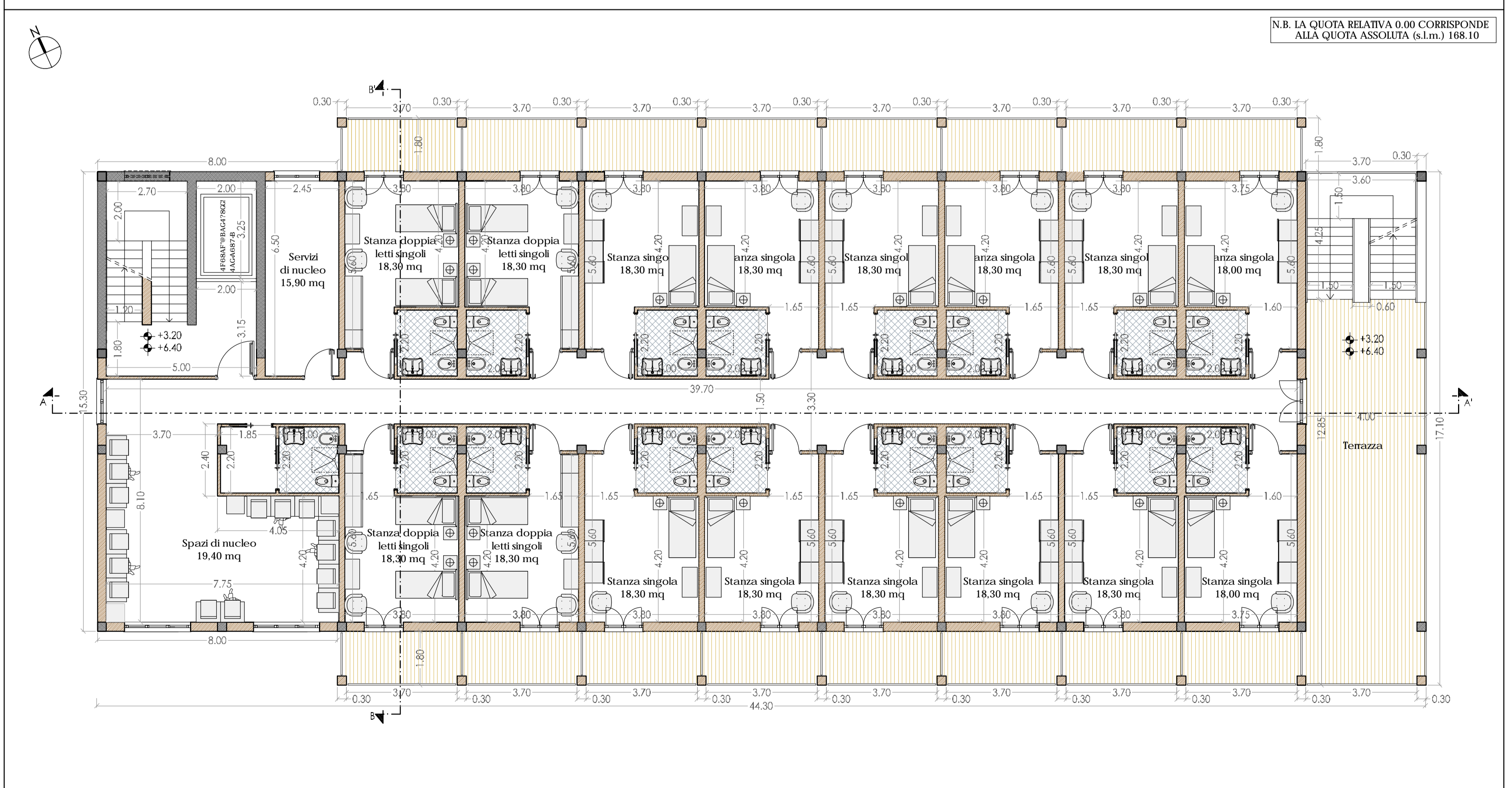
PIANTA PIANO TIPO - rapp. 1:100
