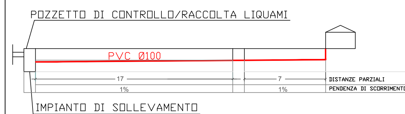
PROFILO LONGITUDINALE - Scarico acque per Nuovi Servizi Igienici (Box Spogliatoio) verso pozzetto di controllo - Scala 1:200
